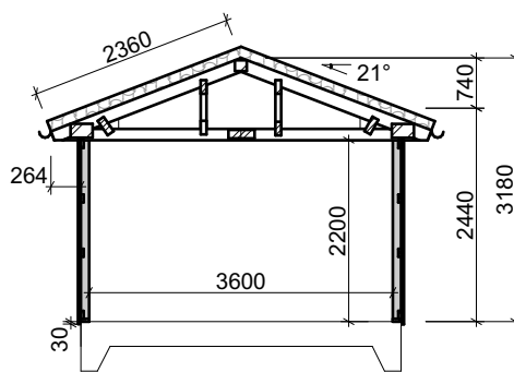
SEKTION A-A
